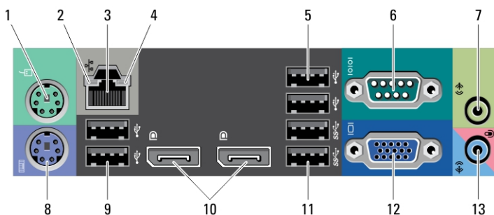
Ilustración 3. Vista del panel posterior de la minitorre y del equipo de escritorio
