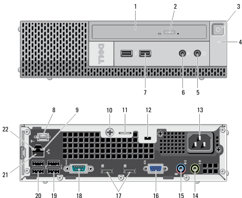
Ilustración 6. Vistas frontal y posterior del factor de forma ultrapequeño
