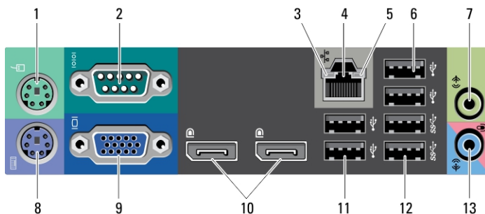
Ilustración 5. Vista del panel posterior del factor de forma pequeño
