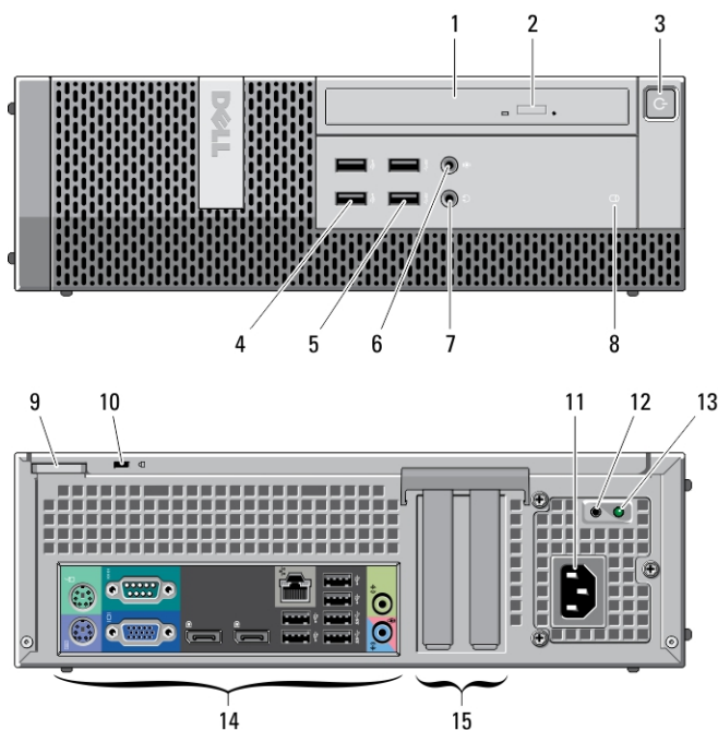
Ilustración 4. Vistas frontal y posterior del factor de forma pequeño
