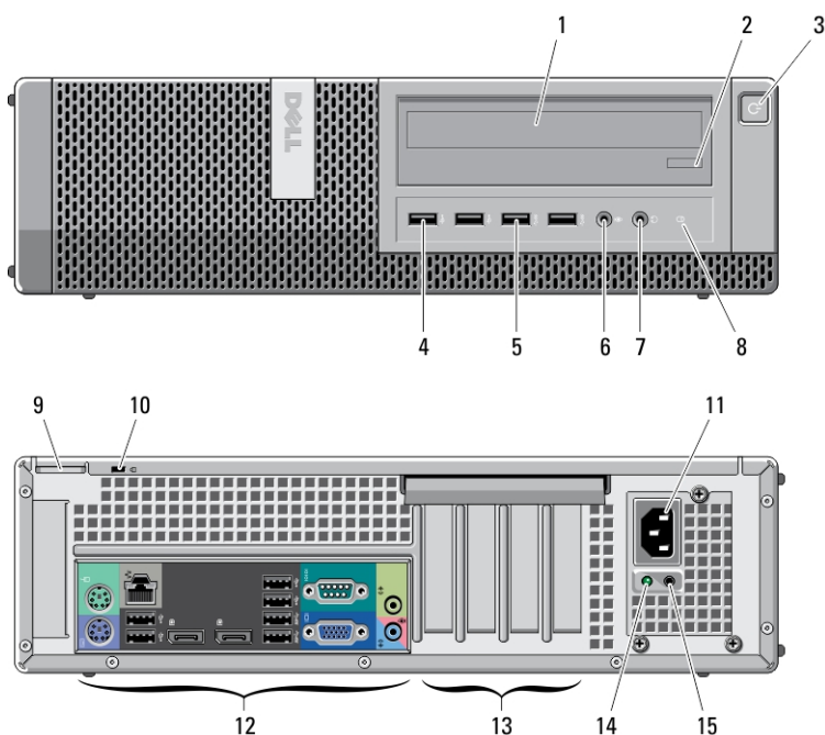
Ilustración 2. Vistas frontal y posterior del equipo de escritorio
